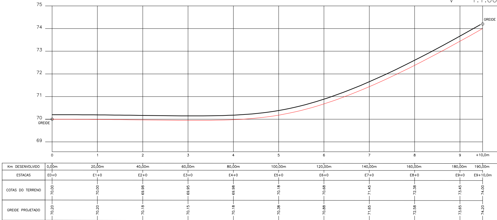
PERFIL DO EIXO LONGITUDINAL DO EIXO–RUA PROJETADA –3 PARAZINHO–RN ESCALAS H– 1:1.000 V– 1:1.00
